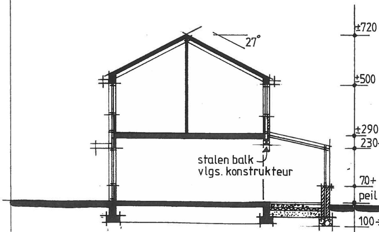
doorsnede
